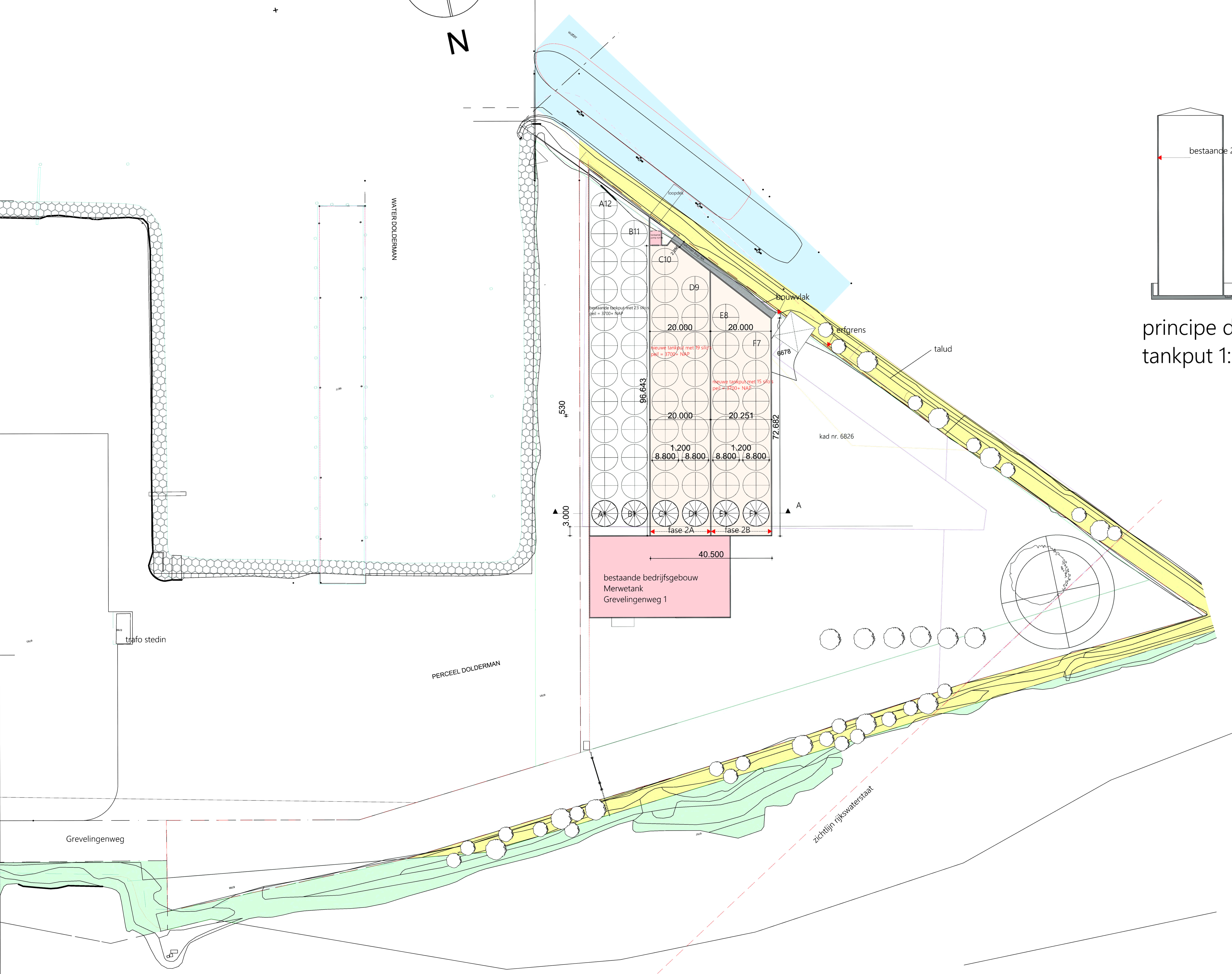
situatie tekening 1: 500
