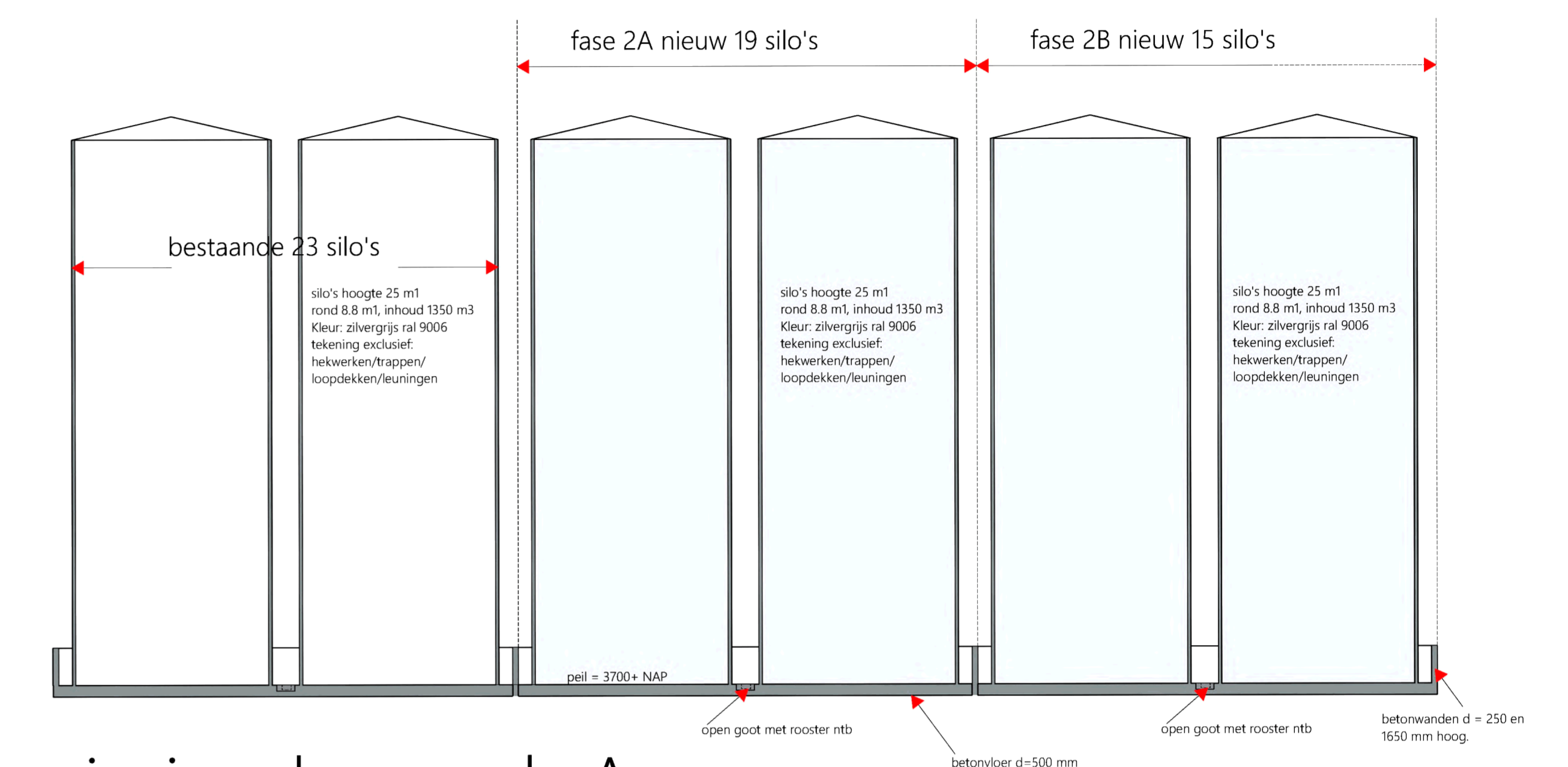
principe doorsnede A tankput 1:200
