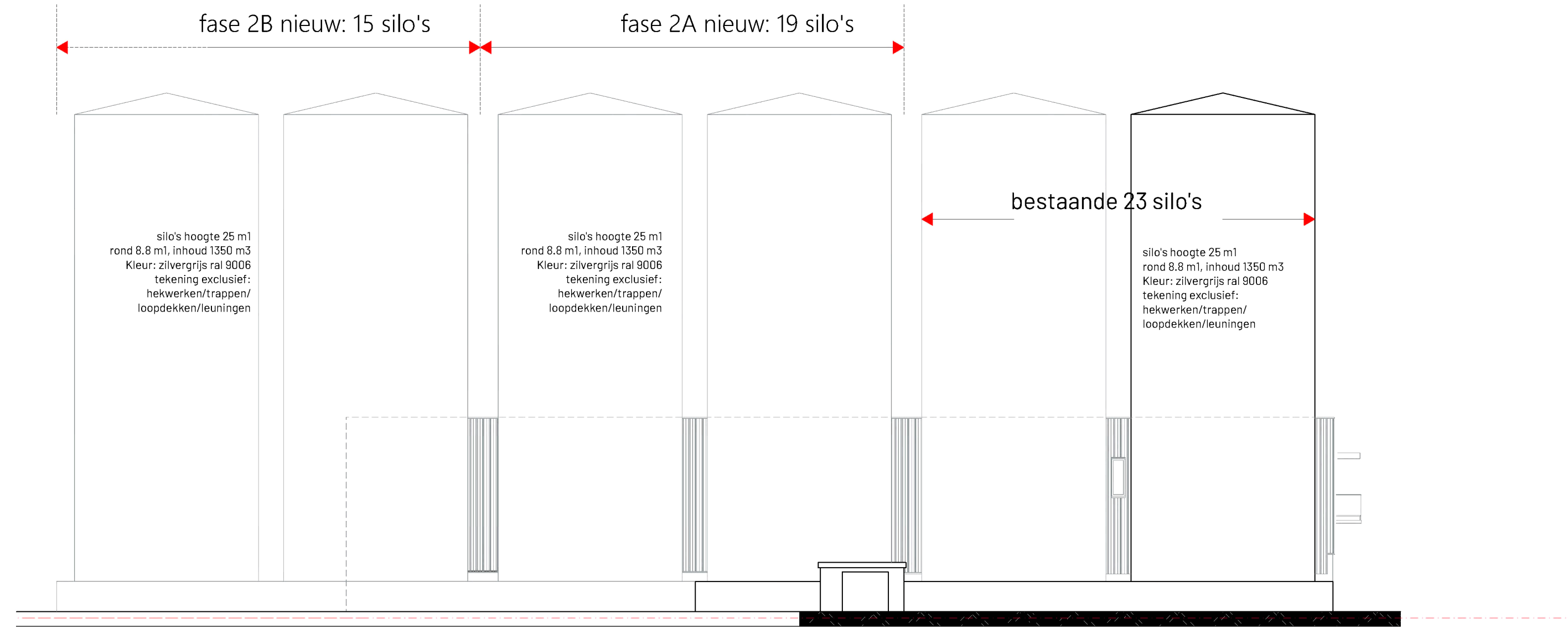
Zuidgevel
