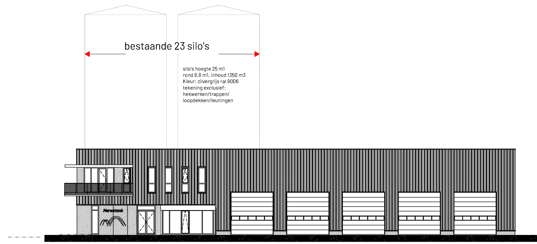
Noordgevel
