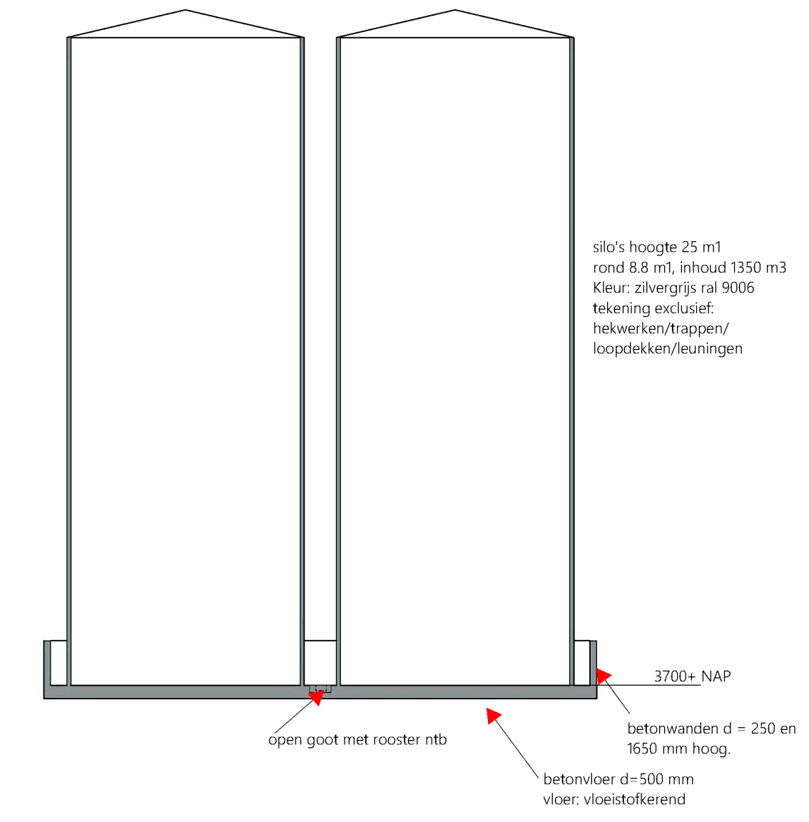
principe doorsnede A tankput 1:200
