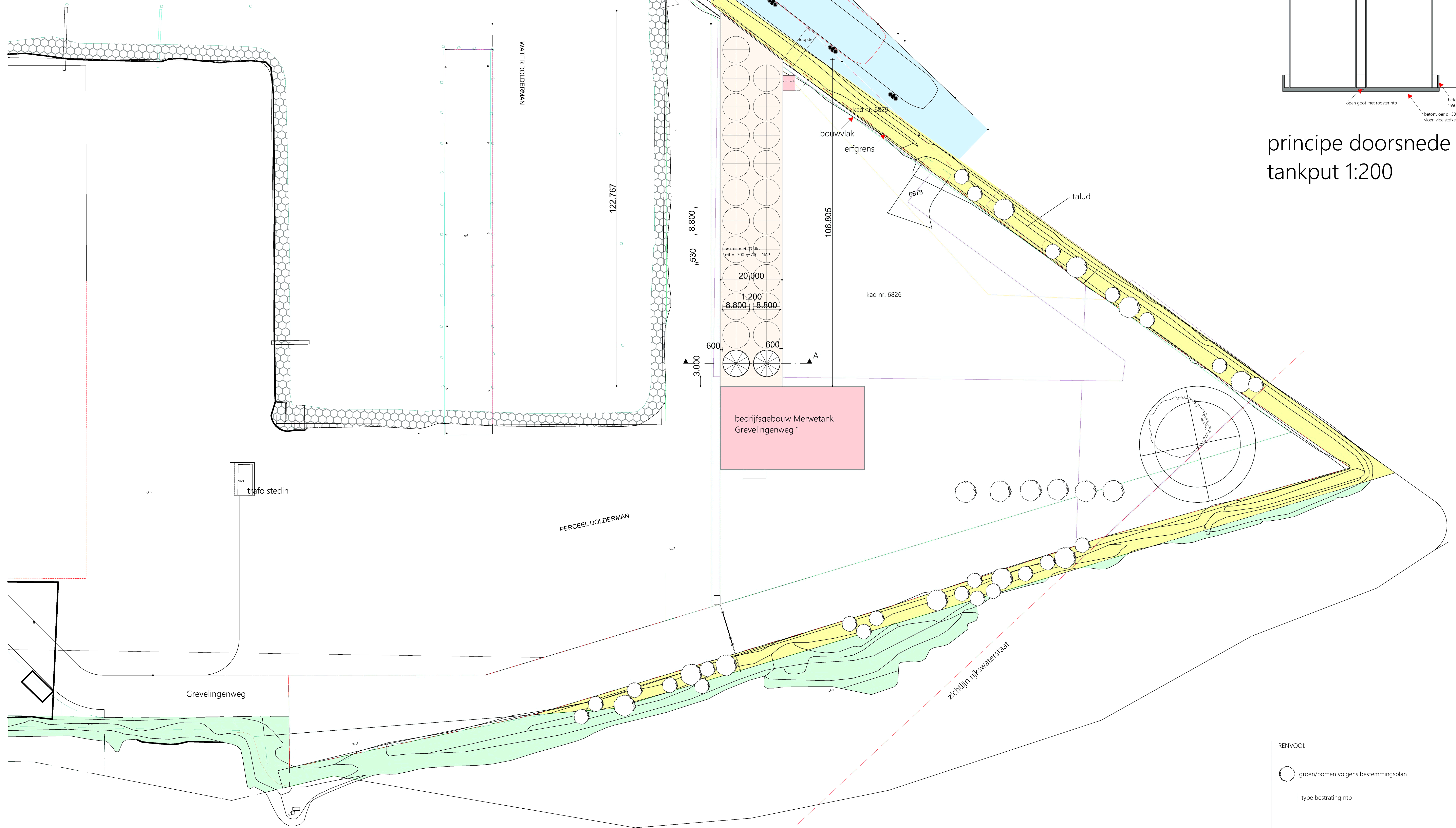
situatie tekening 1: 500
