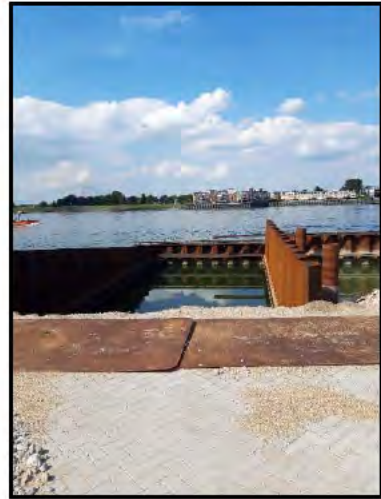
Foto 2: Damwand fase 1, 2 september 2020
