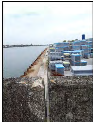
Foto 12: Damwand fase 2, 10 oktober 2022
