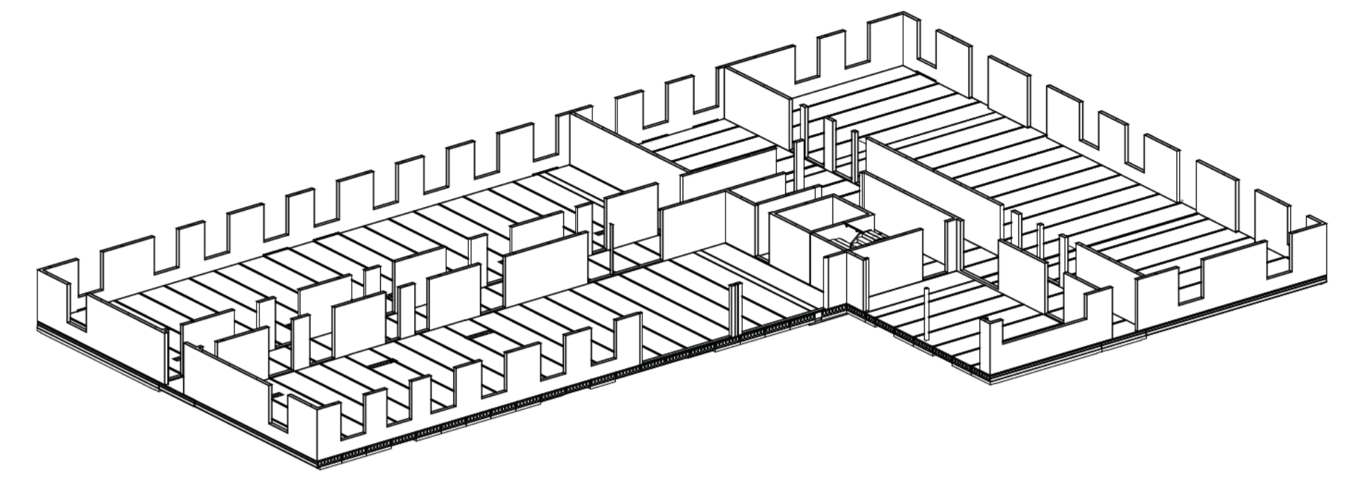
Isometrie Begane grond schaal
